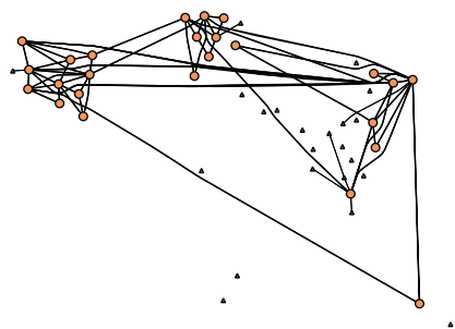
(d) NTT Network: 25 core nodes, 112 uni-direct. links.
